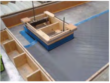
Eksempel på montering af Proofex Engage i støbeformen, hvor elementet har udsparring til eks. vindue/kanal.
